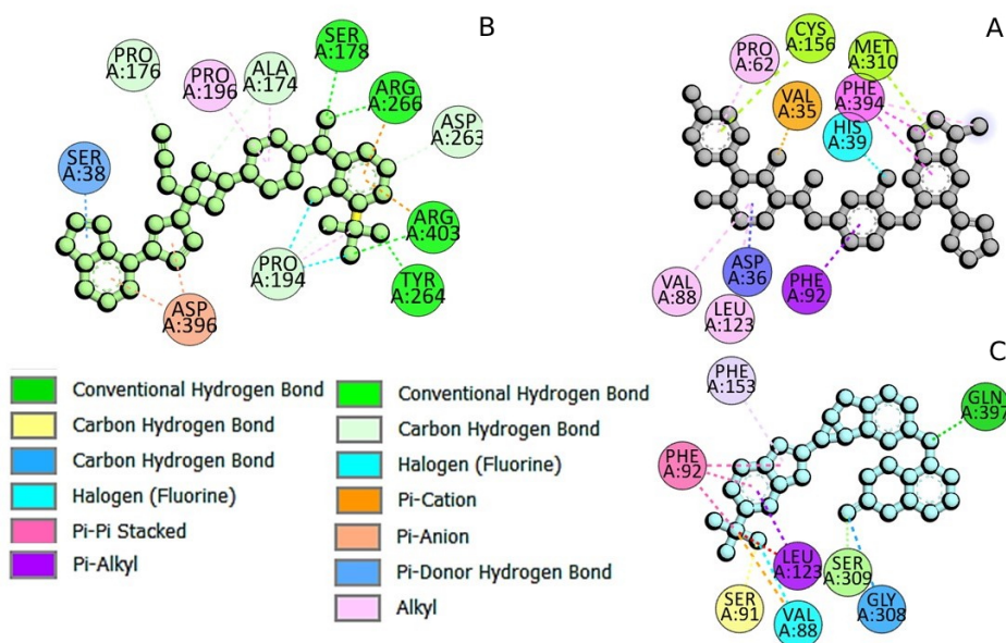
شکل ۱- برهمکنش آنزیم UGT1A1 با A) مرستینیب B) ایٹاسیتینیب C) لیفرافنیب. ساختار لیگاندها در وسط هر تصویر و اسیدآمینوهای آنزیم در اطراف آن نشان داده شده است. برهمکنش ها با نرم افزار دیسکاوری استودیو بررسی و تصویر آن ذخیره شد.
