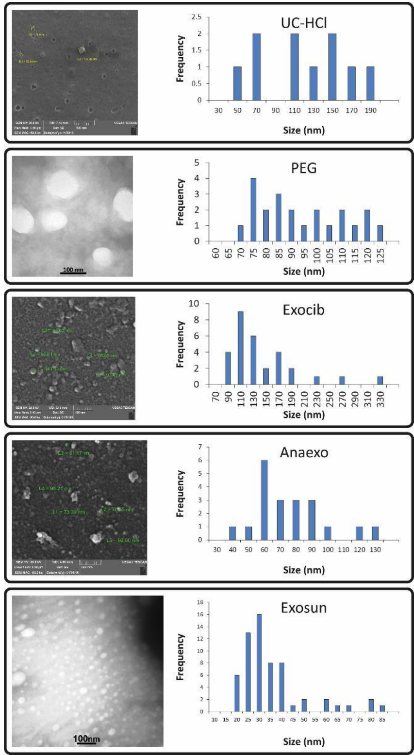
شکل ۵- نمودار پراکندگی سایز ذرات (قطر اگزوزوم برحسب نانومتر) در جداسازی با استفاده از روش‌های مختلف. نمودار اول: UC-HCl، نمودار دوم: PEG، نمودار سوم: Exocib، نمودار چهارم: Anaexo و نمودار پنجم: مربوط به کیت اگزوسان (Exosun) است. در نمودارهای هیستوگرام، فراوانی سایزهای مختلف ذرات اگزوزوم قابل مشاهده است.
