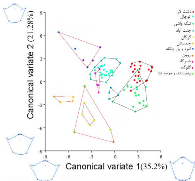
شکل ۶- نمودار تحلیل متغیرهای کانونی (CVA) ریخت‌سنجی هندسی ککسواسترنیت چنگال‌های سمی.
