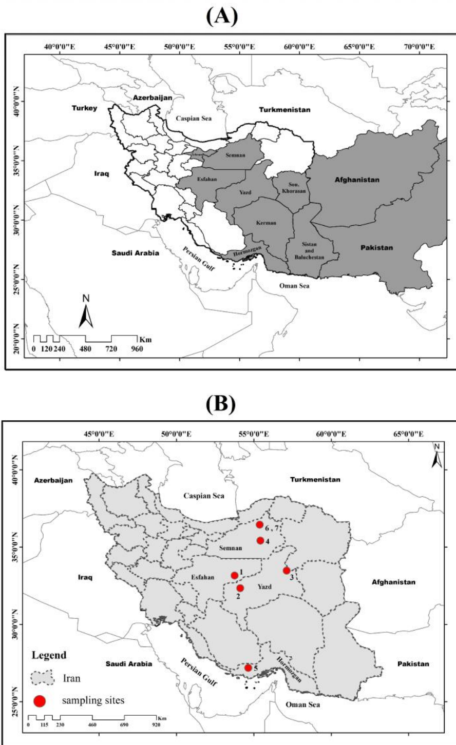
شکل ۱- نقشه پراکنش و نمونه‌برداری Saara asmussi A. نقشه پراکنش جهانی Saara asmussi B. نقشه ایستگاه‌های نمونه برداری Saara asmussi در ایران (۱-نایین، ۲- اردکان، ۳- روستای معظم آباد، ۴- طرود، ۵- بستک، ۶- شاهرود، ۷- شاهرود).
