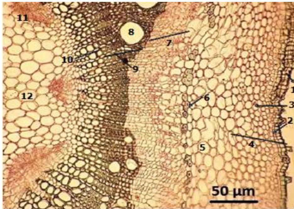
شکل ۴. ساختار تشریحی ریزوم جمعیت نور. ۱- فلم، ۲- فلوژن، ۳- فلودرم، ۴- پریدرم، ۵- پوست نخستین، ۶- اسکله‌تید، ۷- بافت آبکشی، ۸- متاگزیم، ۹- چوب پسین، ۱۰- چوب نخستین، ۱۱- آبکش درونی، ۱۲- مغز پارانشیمی.
