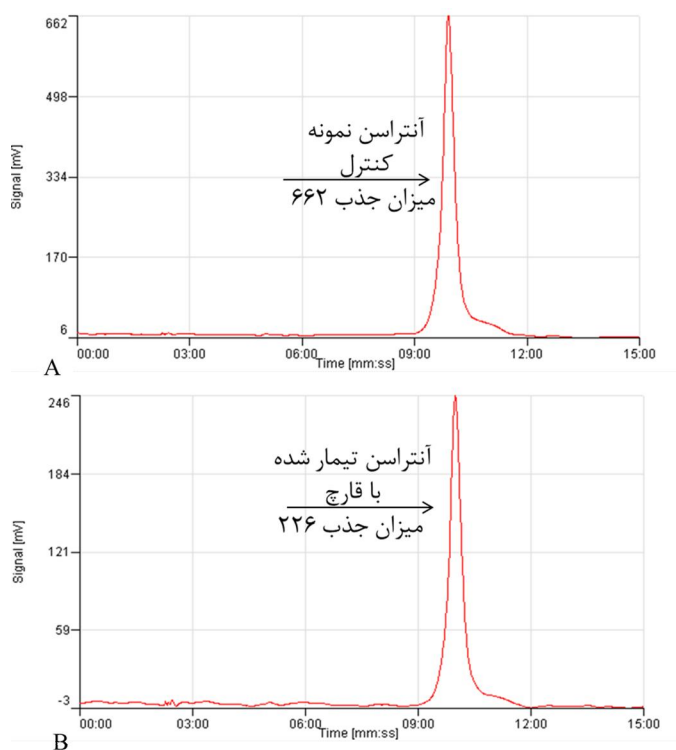
شکل ۴- کروماتوگرام مربوط به حذف آنتراسن A : نمونه شاهد با غلظت ۱۰۰ ppm و B : نمونه پس از تیمار توسط سویه Gliomastix sp. Fig. 4. Anthracene removal chromatogram A : control sample with 100 PPM and B : sample after treatment with Gliomastix sp.
