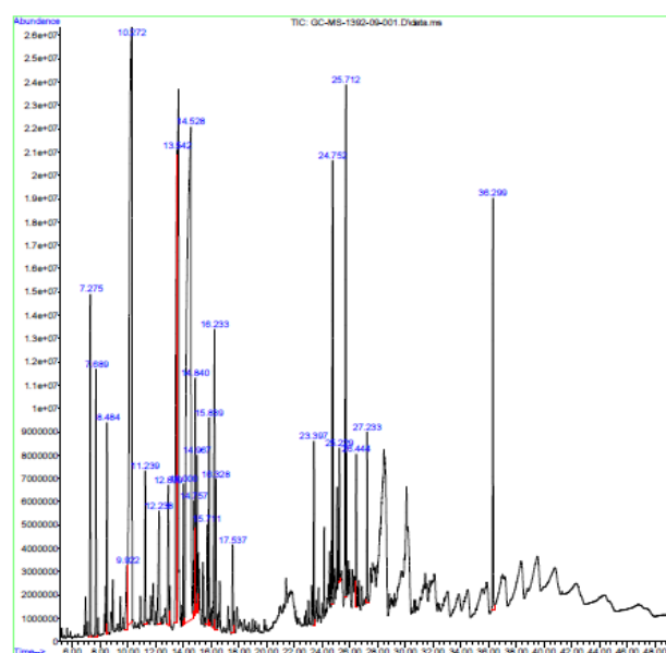
شکل ۲- کروماتوگرام اسانس اسطوخودوس در منطقه بلده.
