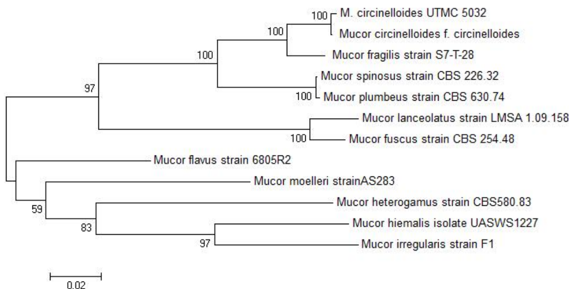
شکل ۳- موقعیت فیلوژنتیکی توالی ژن ITS M. circinelloides UTM 5032. آنالیز اتصال-همسایگی با استفاده از بوت استرپ ۱۰۰۰ پرایمرهای ITS. با الگوریتم اتصال-همسایگی برای هم‌ردیفی و تعیین فاصله‌ی توالی‌ها و نیز نرم‌افزار مگا ۵/۱ نشان می‌دهد.
