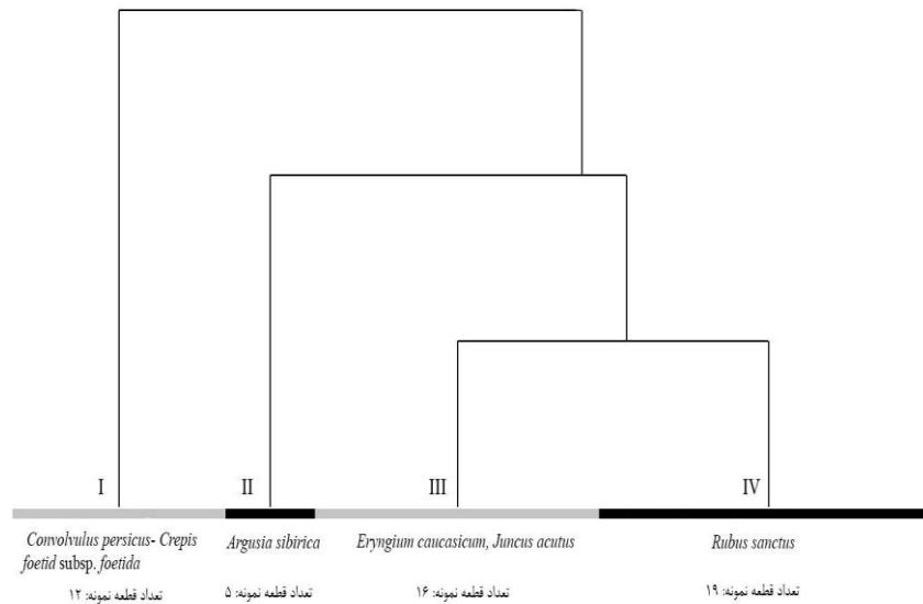
شکل ۳- دندروگرام طبقه بندی قطعات نمونه از طریق Modified TWINSpan.
