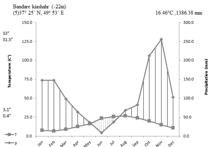
شکل ۲- نمودار منحنی آمبروتیک ایستگاه هواشناسی بندر کیشهر (۲۰۰۷-۲۰۱۲).
