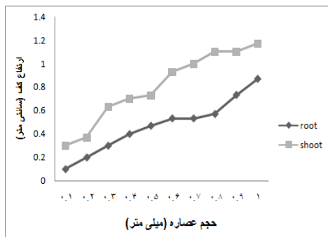
شکل ۲- مقدار کف ایجاد شده براساس غلظت عصاره در گونه Silene spergulifolia . Fig. 2. The amount of formed foam based on extract concentration in Silene spergulifolia .
