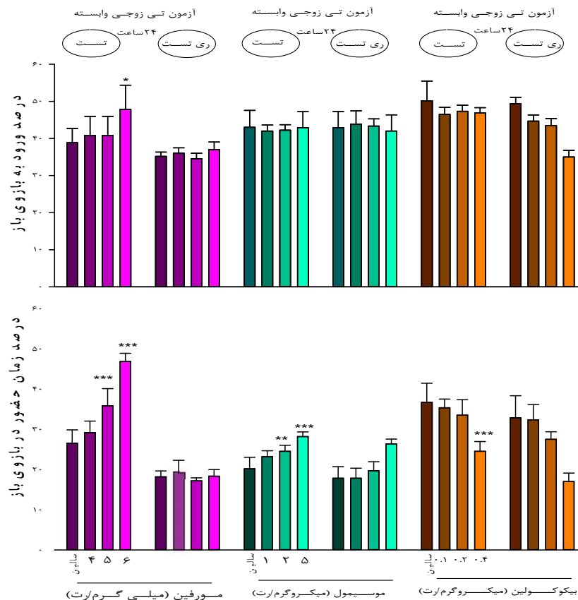
شکل ۱- تاثیر دوزهای مختلف مورفین، موسیمول و بیوکولین روی مقادیر درصد OAT و درصد OAE. علامت * نشان دهنده مقایسه گروه‌های تیمار شده با گروه کنترل سالین P 0.05. علامت ** نشان دهنده مقایسه گروه‌های تیمار شده با گروه کنترل سالین P 0.01. علامت *** نشان دهنده مقایسه گروه‌های تیمار شده با گروه کنترل سالین P 0.001.
