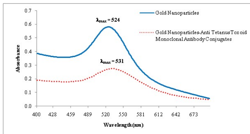
شکل ۳- طیف LSPR تأیید کننده کانجوگاسیون نانوذرات طلا-آنتی بادی مونوکلونال ضد توکسوئید کزاز؛ طیف LSPR نانوذرات کلونیدی ۱۰ نانومتر یک \lambda_{max} برابر با ۵۲۴ نانومتر (خط ممتد آبی) نشان می‌دهد و پس از کانجوگه شدن با آنتی بادی \lambda_{max} به میزان ۷ نانومتر به سمت راست جابه‌جا می‌شود (خط نقطه چین قرمز).
